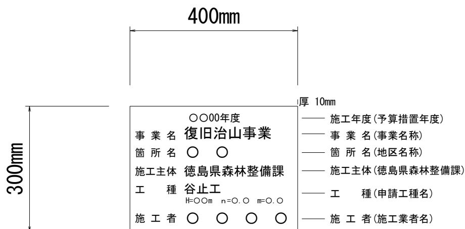
図1 銘板の寸法及び記載事項
